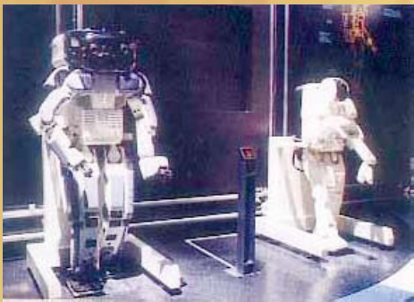
我国第一台类人型机器人“中国先行者”
